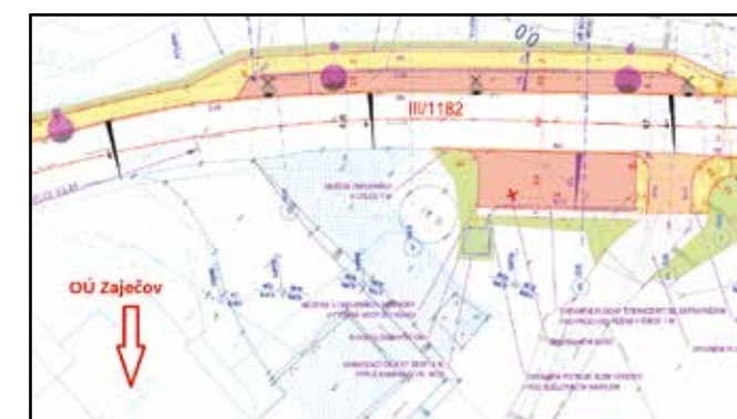
Parkoviště u hasičské zbrojnice – Situační výkres
